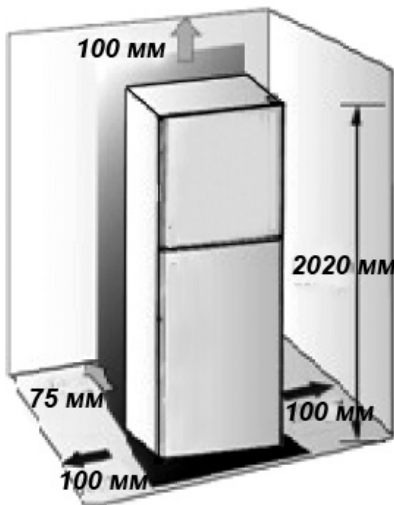
Рисунок-схема рекомендуемого размещения холодильника
