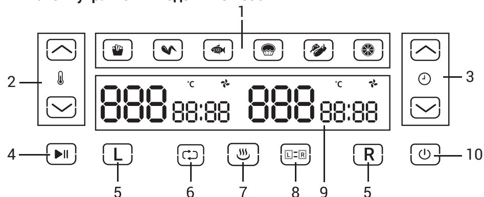
Панель управления модели MGD 900 B
