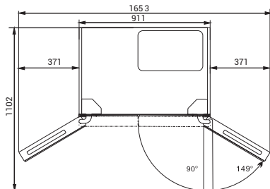
RFQ-550DX NFGB / GW inverter
